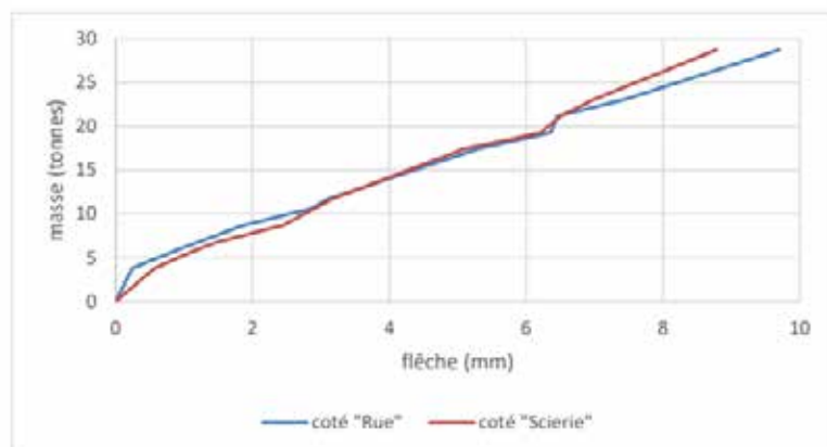
Figure 5 : Évolution de la flèche centrale par rapport à la charge
